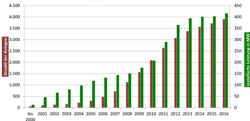
Entwicklung der Anzahl von Erneuerbare-Energien-Anlagen und der installierten Leistungen im Landkreis Bautzen von 2000 bis 2016
